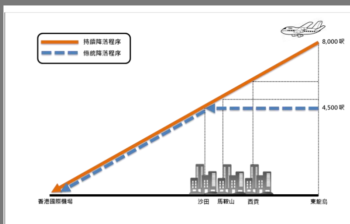
圖 2-2：持續降落程序示意圖
