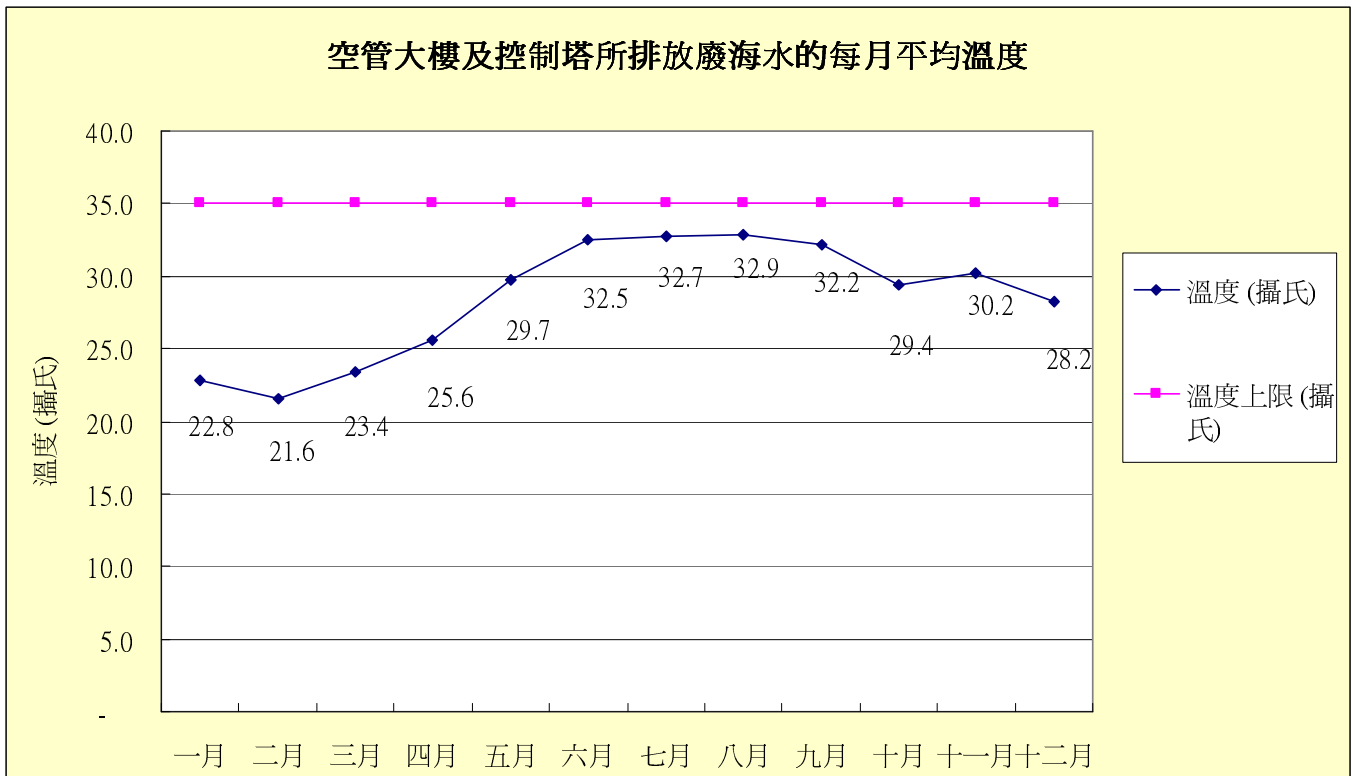
圖十七：空管大樓及控制塔所排放廢海水的每月平均溫度
