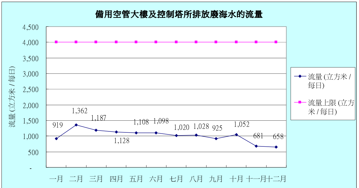
圖十六：備用空管大樓及控制塔所排放廢海水的每日平均流量
