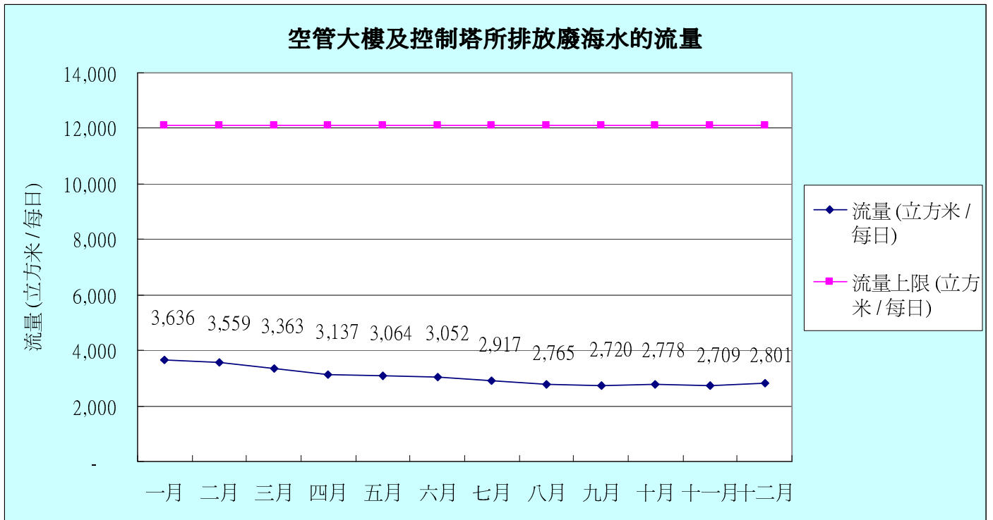
圖十五：空管大樓及控制塔所排放廢海水的每日平均流量
